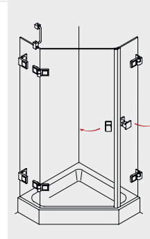
MIDRA 259 Fünfeckdusche mit 2 Drehtüren
