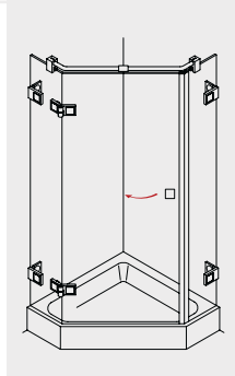
MIDRA 255 Fünfeckdusche mit 1 Drehtür
