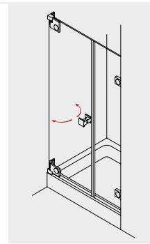
TIBA 110 Pendeltür und Fixteil in Nische
