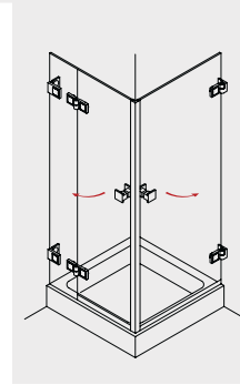
MIDRA 239 Drehtür am Fixteil und Drehtür an der Wand als Ecklösung
