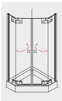
TIBA 250 Fünfeckdusche mit 2 Pendeltüren
