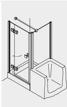
KANO 231 Drehtür am Fixteil mit verkürzter Seitenwand
