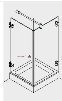
ARANO 130 Drehtür mit Seitenwand
