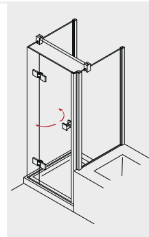
PADEA 234 U-Kabine mit Pendeltür und verkürzter Seitenwand
