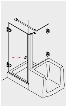
ARANO 131 Drehtür mit verkürzter Seitenwand
