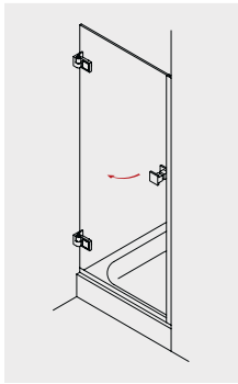
MIDRA 100 Drehtür in Nische
