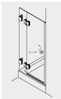
PERA 200 Drehtür am Fixteil in Nische
