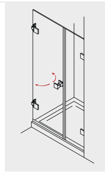
PADEA 110 Pendeltür und Fixteil in Nische
