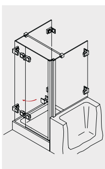
KANO 234 U-Kabine mit Drehtür und verkürzter Seitenwand
