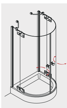
TIBA 263 Halbkreisdu- sche mit 2 Pendeltüren
