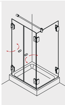
NORMA 135 2 Pendeltüren mit Seitenwand
