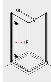
MIDRA 230 Drehtür am Fixteil mit Seitenwand
