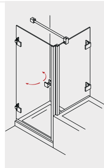
PADEA 131 Pendeltür mit verkürzter Seitenwand
