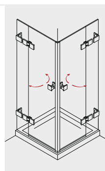
PADEA 220 EckEinstieg mit 2 Pendeltüren an Fixteilen
