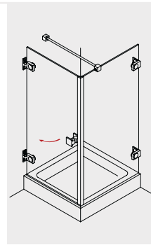
KANO 130 Drehtür mit Seitenwand
