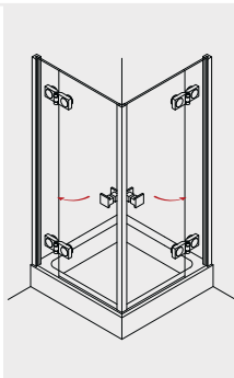
KANO 220 EckEinstieg mit 2 Drehtüren an Fixteilen
