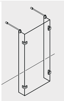
TYP 520 mit Wandwinkeln
