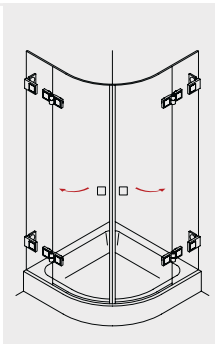
MIDRA 260 Viertelkreis- dusche mit 2 Drehtüren
