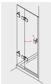
PADEA 200 Pendeltür am Fixteil in Nische
