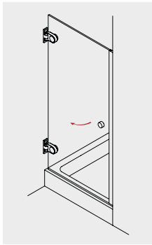
ARANO 100 Drehtür in Nische
