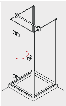
PADEA 233 U-Kabine mit Pendeltür
