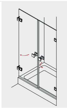
MIDRA 105 2 Drehtüren in Nische
