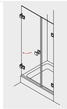
MIDRA 110 Drehtür und Fixteil in Nische
