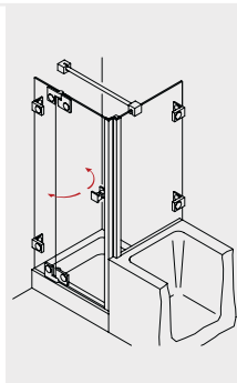
TIBA 231 Pendeltür am Fixteil mit verkürzter Seitenwand
