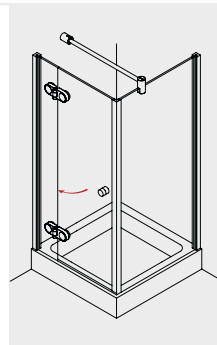
ARANO 230 Drehtür am Fixteil mit Seitenwand
