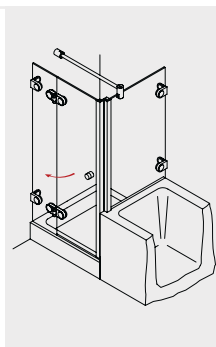
ARANO 231 Drehtür am Fixteil mit verkürzter Seitenwand
