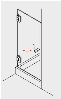
NORMA 100 Pendeltür in Nische
