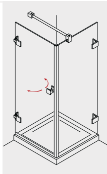
PADEA 130 Pendeltür mit Seitenwand
