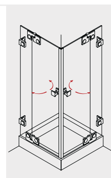
TIBA 220 EckEinstieg mit 2 Pendeltüren an Fixteilen
