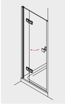
MIDRA 200 Drehtür am Fixteil in Nische
