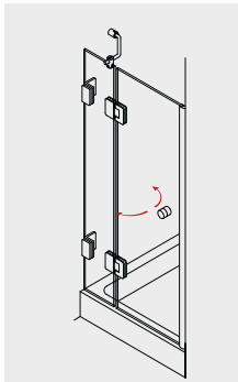
NORMA 200 Pendeltür am Fixteil in Nische
