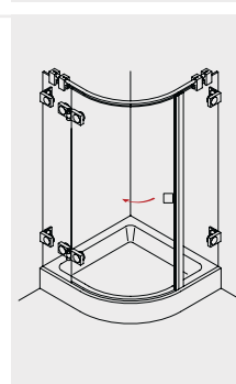
KANO 265 Viertelkreis- dusche mit 1 Drehtür
