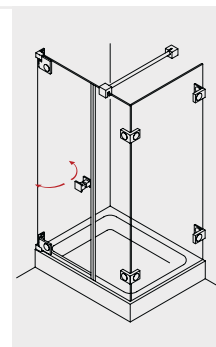
TIBA 140 Pendeltür und Fixteil mit Seitenwand
