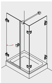
MIDRA 140 Drehtür und Fixteil mit Seitenwand
