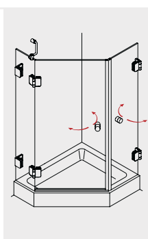
PERA 259 Fünfeckdusche mit 2 Drehtüren
