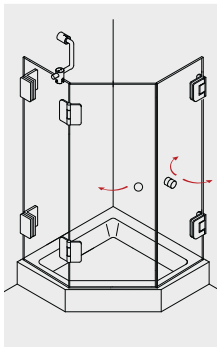
NORMA 259 Fünfeckdusche mit 1 Drehtür und 1 Pendeltür
