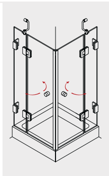
NORMA 220 Eck Einstieg mit 2 Pendeltüren an Fixteilen
