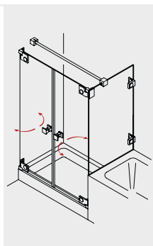
TIBA 136 2 Pendeltüren mit verkürzter Seitenwand
