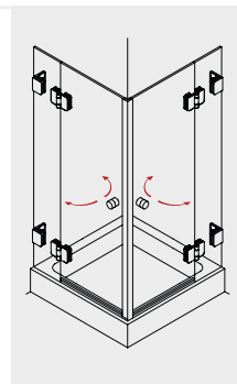
PERA 220 EckEinstieg mit 2 Drehtüren an Fixteilen
