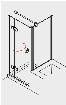
PADEA 231 Pendeltür am Fixteil mit verkürzter Seitenwand
