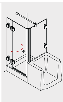
PERA 230 Drehtür am Fixteil mit Seitenwand
