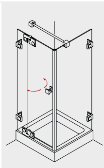
TIBA 230 Pendeltür am Fixteil mit Seitenwand
