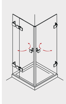
PADEA 239 Pendeltür am Fixteil, Pendeltür an der Wand als Ecklösung
