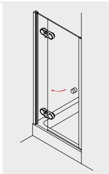
ARANO 200 Drehtür am Fixteil in Nische
