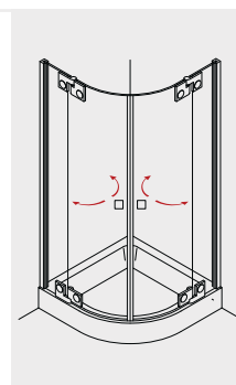
TIBA 260 Viertelkreis- dusche mit 2 Pendeltüren
