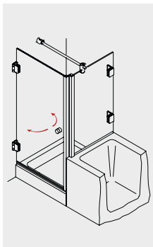
PERA 131 Drehtür mit verkürzter Seitenwand
