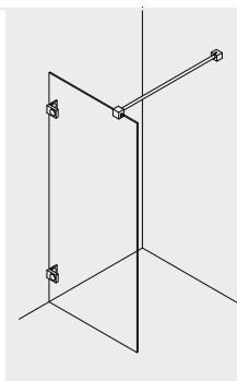
TYP 500 mit Wandwinkeln
